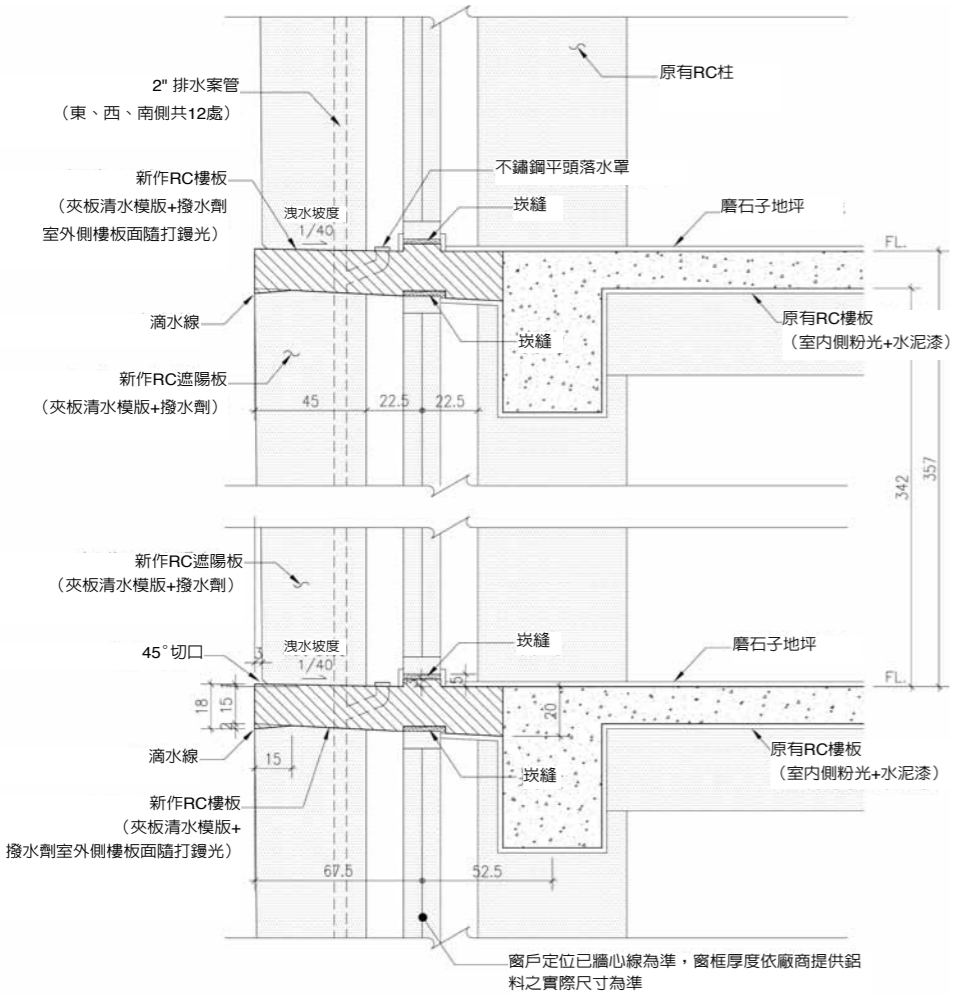
B棟雨遮樓版剖面標準圖 Scale = 1/60
